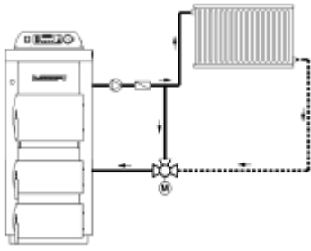
Рис. 7а. Зразок монтажу змішувального клапана в інсталяції з регулюванням кількості (оберігає котел від «холодного» повернення теплоносія)
