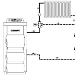
Рис.7б. Зразок монтажу змішувального клапана в інсталяції з регулюванням якості (не оберігає котел від «холодного» повернення теплоносія)
