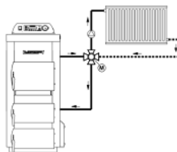
Рис. 6а. Зразок монтажу змішувального чотириходового клапана
