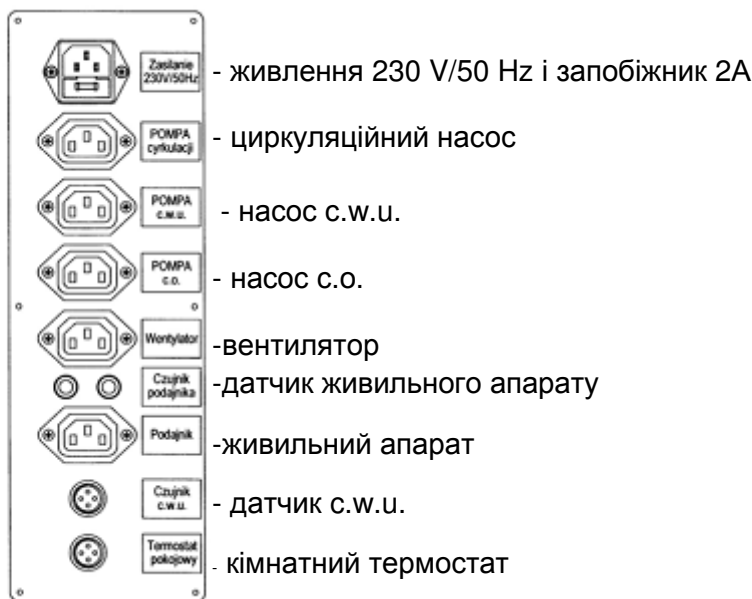
Рис.5. Стінка під'єднання
