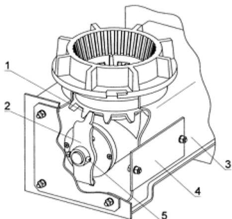
Рис. 12. Оборотна колосникова решітка
