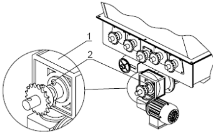
Рис. 4. Вал живильного апарату зі шплінтом:
