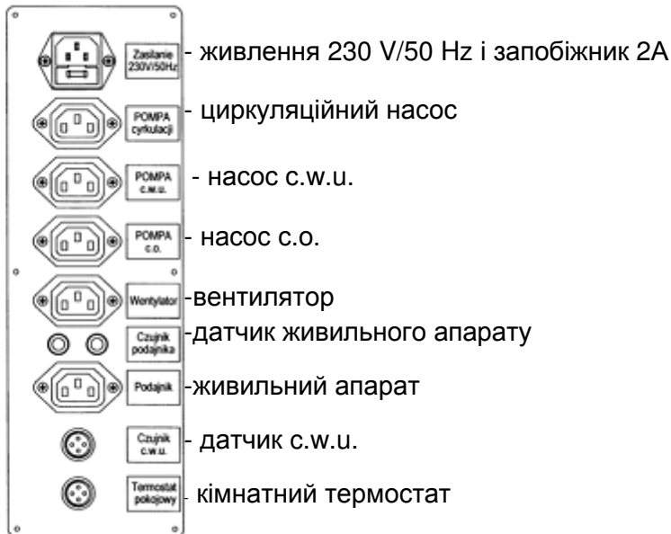
Рис. 13. Стінка під'єднання
