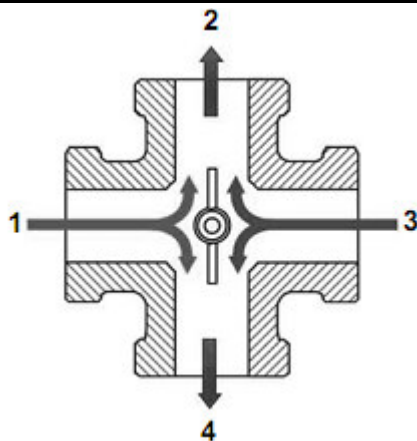
Рис. 6. Чотириходовий змішувальний клапан
