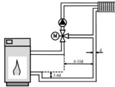
Зразок монтажу змішувального клапана
