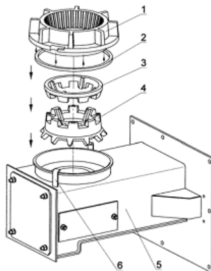
Рис. 2. Оборотна колосникова решітка:
